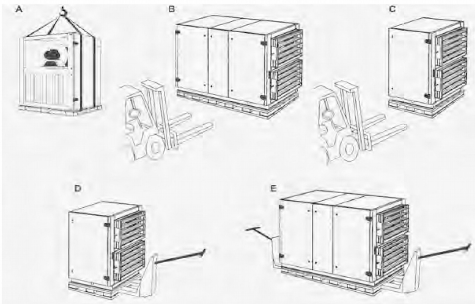
Рисунок 1 Способы транспортировки
