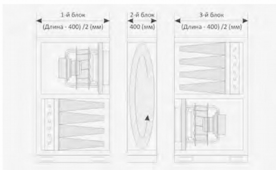
Рисунок 3 Секции установки
